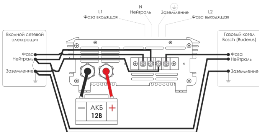
Схема подключения ИБПС к газовому котлу Bosch (Buderus)
